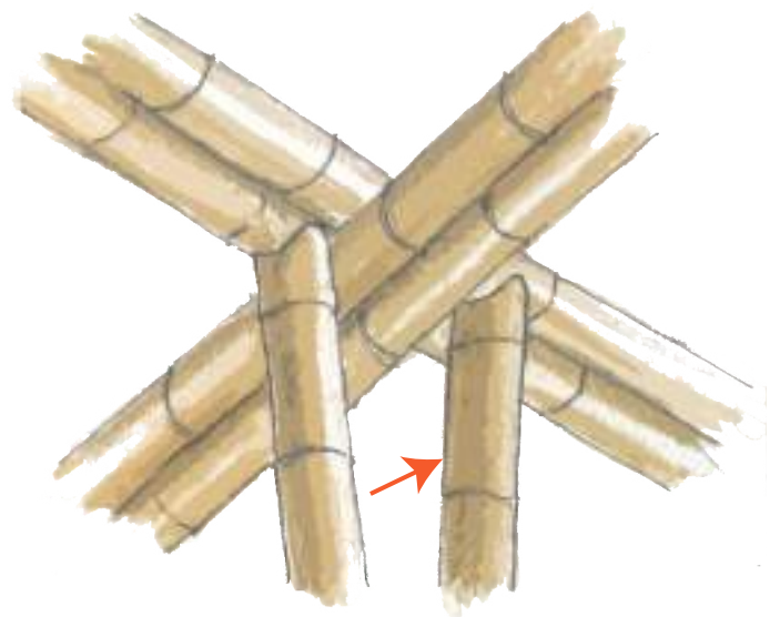
2. Culmos soportando un culmo diferente del segundo nivel de correas.
