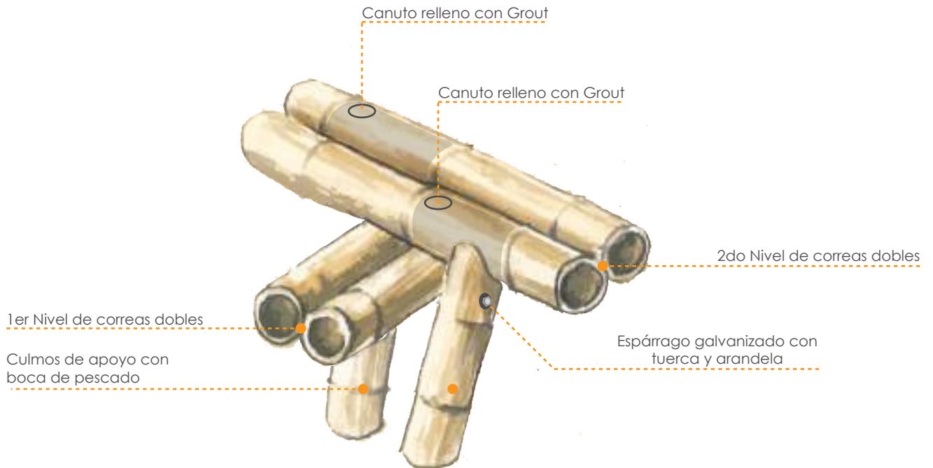
Unión Culmos con correas dobles Vista Frontal
