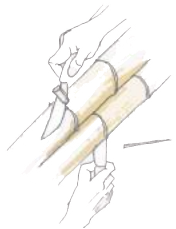
C) Recortar los extremos que sobresalgan de la correa, utilizando una següeta y un cuchillo para afinar el corte.
