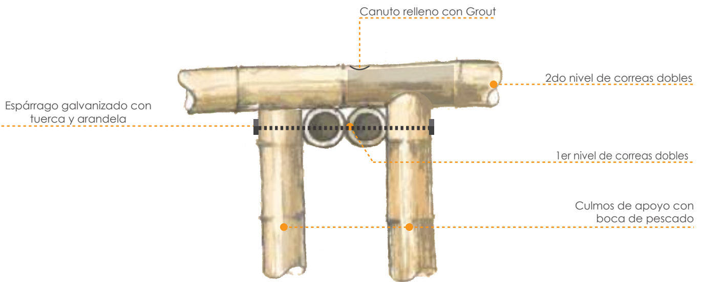
Unión Culmos con correas dobles Vista Frontal
