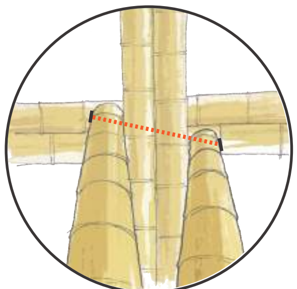
Unión Culmos con correas dobles Vista desde abajo
