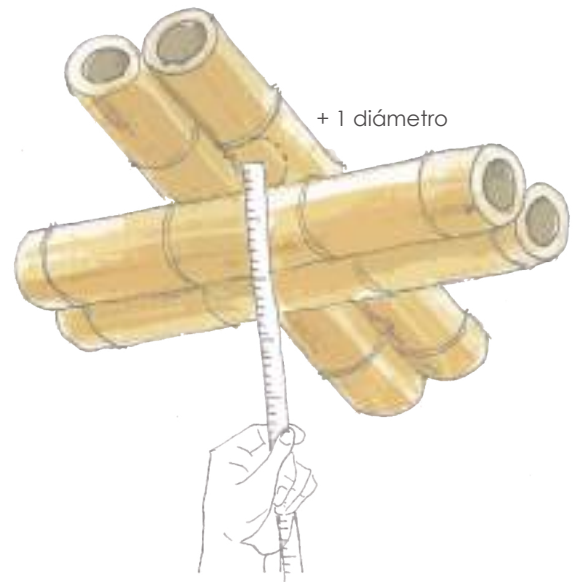
Medida en correas del paraboloides
