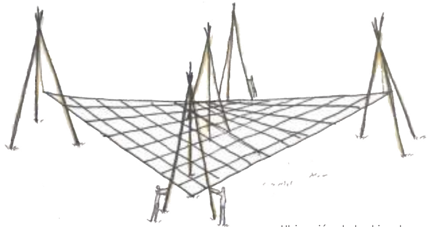
Ubicación de los trípodes
