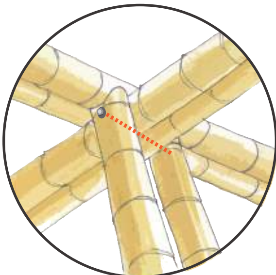
Unión Culmos con correas dobles Vista en perspectiva
