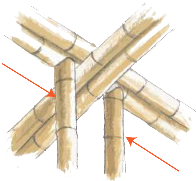
1. Culmos abrazando primer nivel de correas dobles
