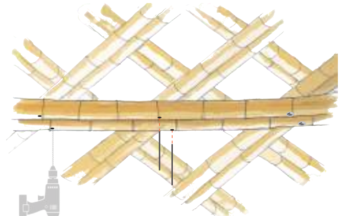
Unión de correa doble a estructura del paraboloide
